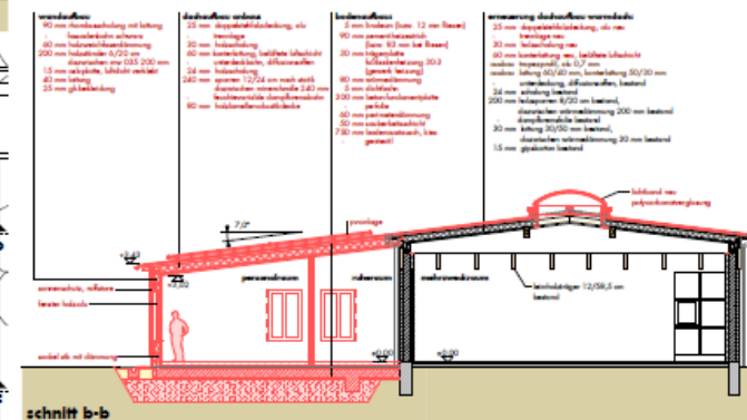
schnitt b-b
