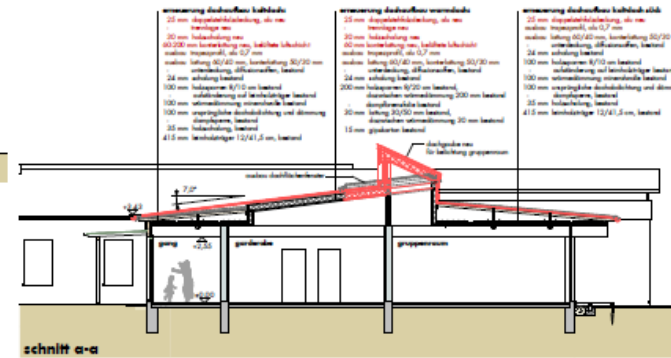
schnitt a-a
