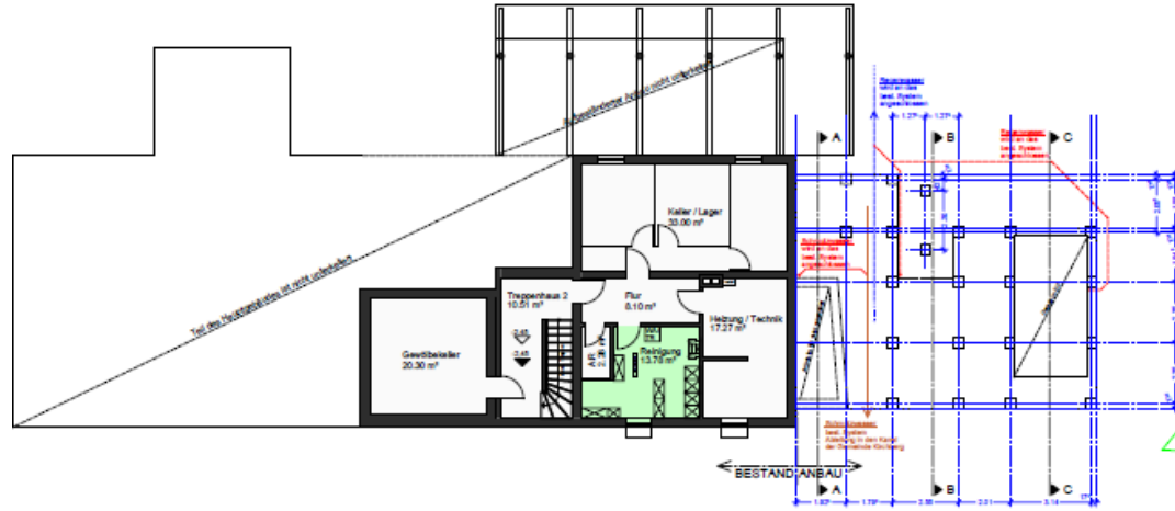
Kellergeschoss
